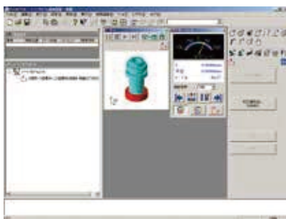
▲ 主界面
